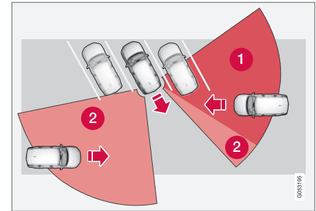
В ъгловото място за паркиране Cross Traffic Alert може да е напълно „сляпа“ от едната страна.
