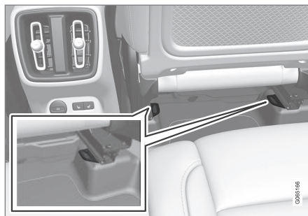
Местоположения на точки за монтаж в задната седалка.
