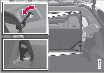
Arkaya takma.
