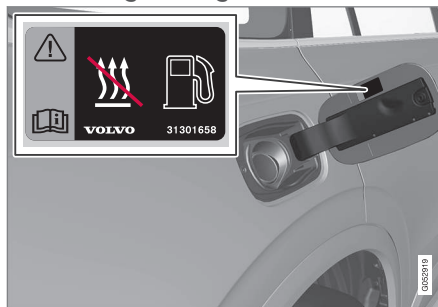
Varselmerke på tanklokkkluken.
