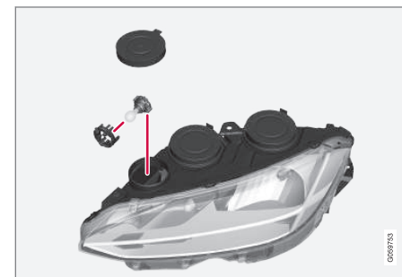
Ляв преден фар.
