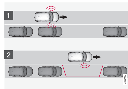
Procédure de recherche avant le stationnement parallèle.
