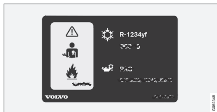
2 Πινακίδα για σύστημα A/C, για αυτοκίνητα με ψυκτικό R1234yf.
