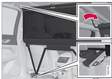
Преден монтаж.
