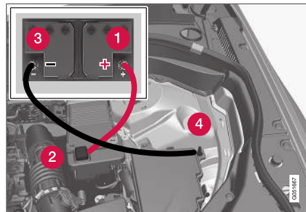
Käynnistyskaapeliin kiinnityspisteet.
