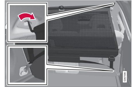
Montaje trasero.
