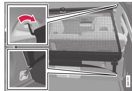
Montaje trasero.
