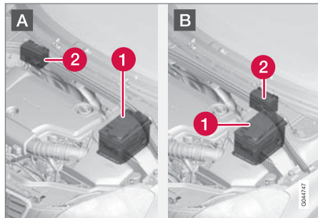
A: سيارة ذات عجلة قيادة يسرى. B: سيارة ذات عجلة قيادة يمينى.
