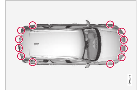
Emplacement des capteurs d'aide au stationnement 126 .
