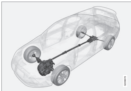
Principeschets AWD 7 .
