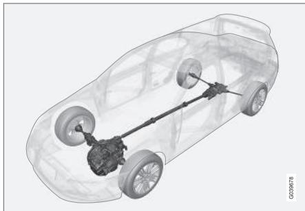
Zasada działania napędu AWD 7 .
