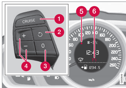
Przyciski przy kierownicy i wyświetlacz w samochodach bez ogranicznika prędkości 6 .
