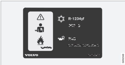
2 Letrero del sistema A/C en vehículos con el fluido refrigerante R1234yf.
