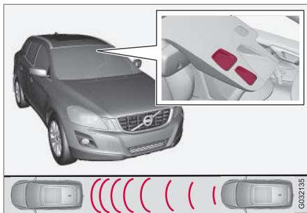
Vysílač a přijímač laserového senzoru v čelním okně 17 .
