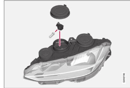
좌측 전조등.
