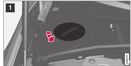
냉각수 탱크, 좌측 운전 차량.
