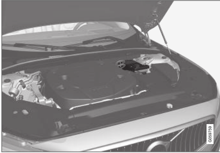
보조 배터리는 스트럿 타워 옆의 박스에 있습니다.
