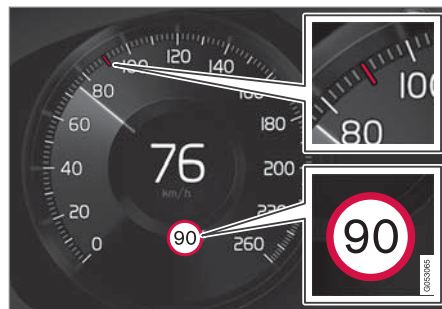
記録された速度情報の例 82
