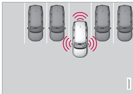
Αρχή λειτουργίας για την τοποθέτηση του αυτοκινήτου κατά την κάθετη στάθμευση.
