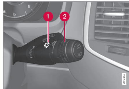
Правий перемикач на колонці рульового управління.
