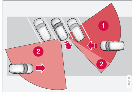
Açılı bir park alanında CTA tek tarafa tamamen "kör" olabilir.
