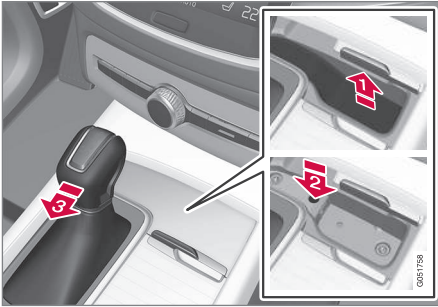
Översikt över stor växelspak.
