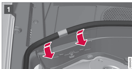
Expansionskärlet för kylsystem
