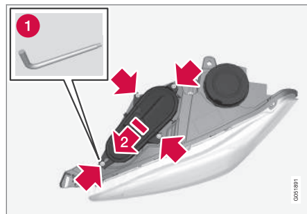
Linker koplamp.
