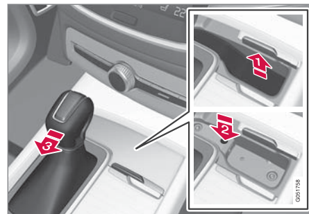
大型セレクトーレバーの概観
