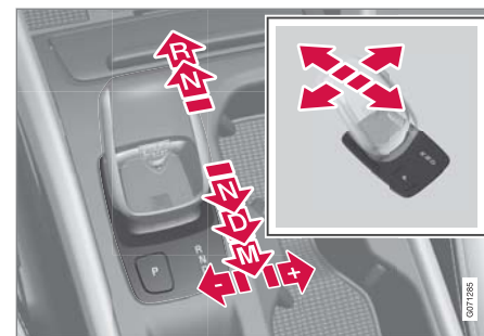
小型セレクトターレバーとギヤ位置の概観
