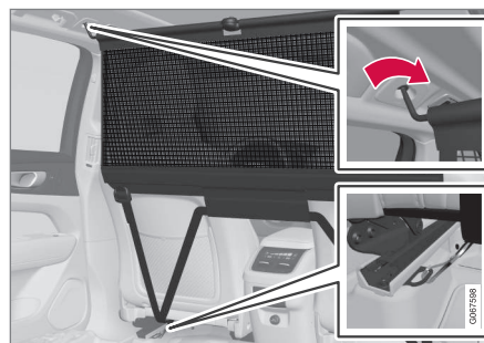
Монтаж впереди.
