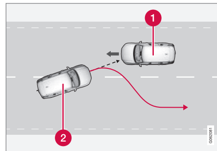
A função pode assistir dirigindo de volta para a sua faixa de rodagem.
