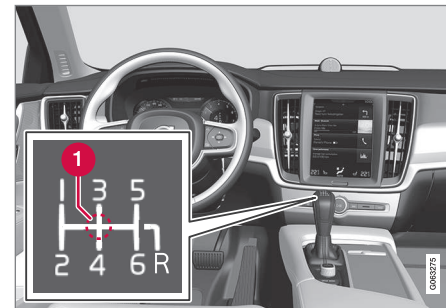
Übersicht über Wählhebel und Schaltmuster.
