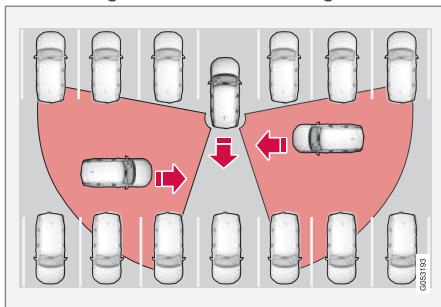
Bereich, in dem die Funktion CTA Hindernisse beim Zurücksetzen erkennen kann.
