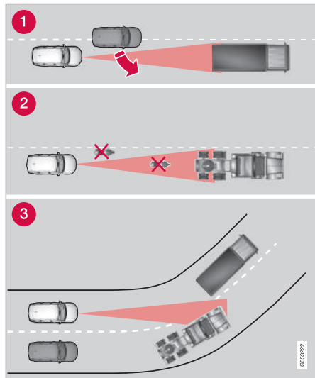
Radarenhedens synsfelt
