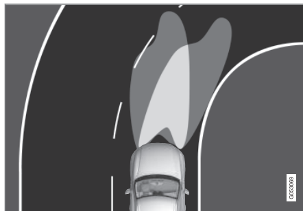
Nivelamento dos faróis com a função desativada (esquerda) e ativada (direita).
