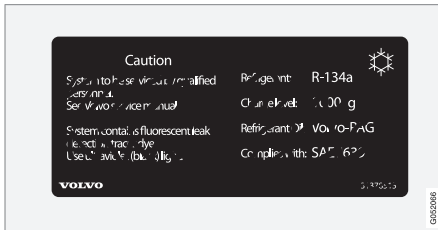
2 Πλακίδια συστήματος A/C για αυτοκίνητα με ψυκτικό R134a.
