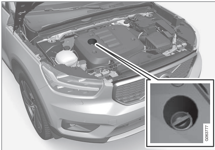
Einfüllrohr 12/13
