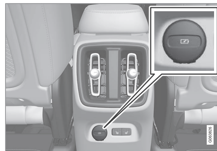
Intrare USB* (tip C) în capătul spate al consolei tunel pentru încărcarea telefoanelor și tabletelor, de exemplu 8 .
