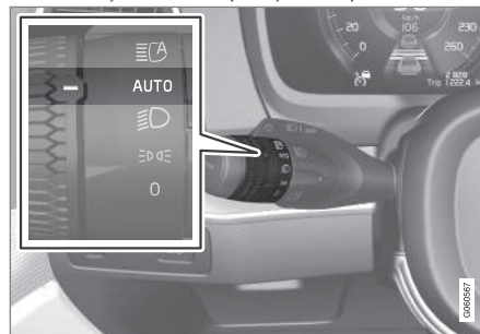
Inelul rotativ al comutatorului manetei în poziția AUTO .
