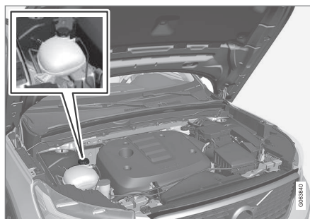
Vasul de expansiune pentru lichidul de răcire
