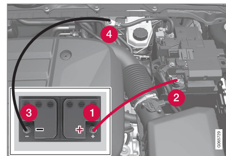
Punctele de fixare pentru cablurile de alimentare.
