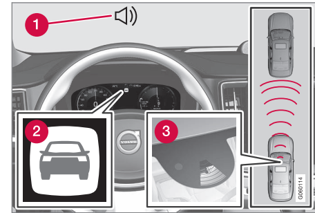
Elementy układu
