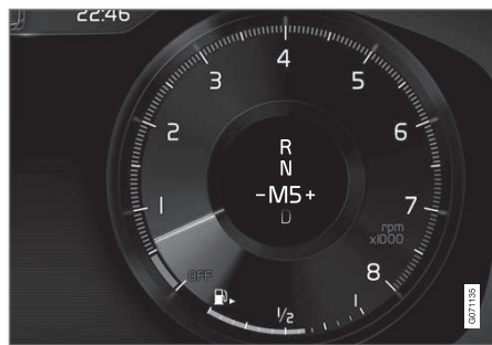
Display del conducente in caso di cambio marce con le leve al volante in modalità di cambio manuale.
