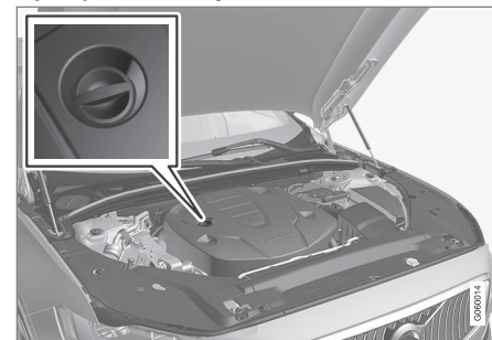
Påfyllningsrör 112
