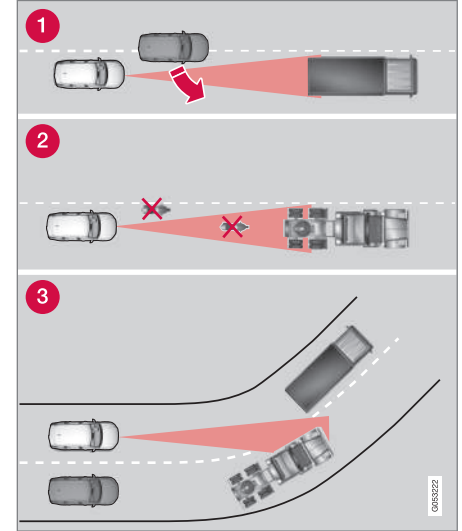
Radar ünitesinin görüş alanı
