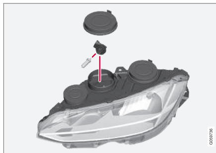
Faro sinistro.
