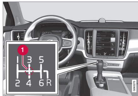
Panoramica della leva selettore e schema di cambio.
