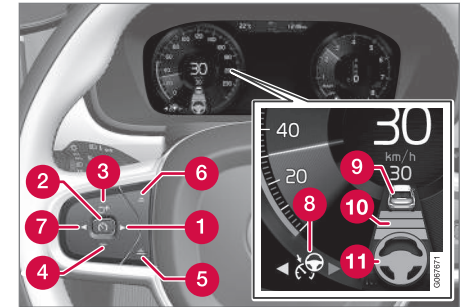
A funkció gombjai és szimbólumai.
