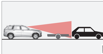
Χαμηλό ρυμουλκούμενο στη σκιά του ραντάρ
