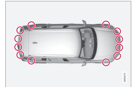
Emplacement des capteurs d'aide au stationnement
