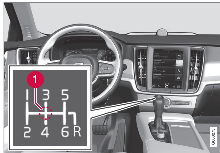
Käigukangi ja käigumustrite ülevaade.
