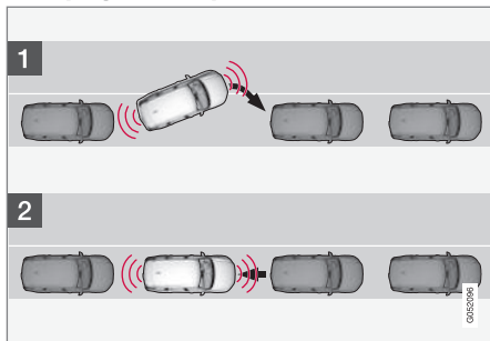
Paigutamise põhimõte paralleelsel parkimisel.
