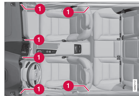
Amplasarea gurilor de aer în habitacul.
