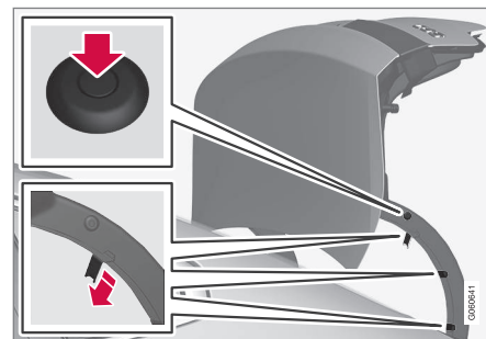
Пластмассовая защита петель крепится с помощью одной пластмассовой заклепки и трех защелок.
