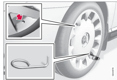
ホイールボルトのプラスチックキャップ取り外しツール
