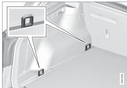
カーゴスペースの固定ポイント位置
