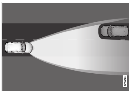
Função adaptativa: Médios direcionados para o veículo em sentido contrário, mas com máximos em ambos os lados do veículo.
