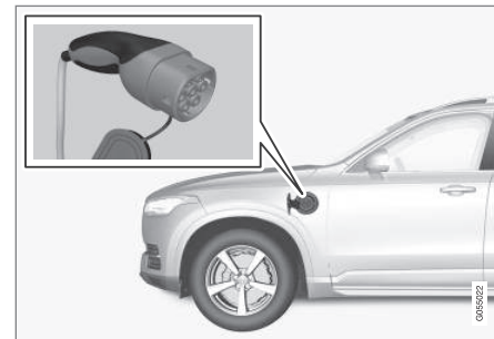
Uchwyt przewodu ładującego i gniazdo do ładowania.
