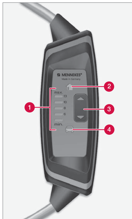
控制箱指示器及控制裝置。
