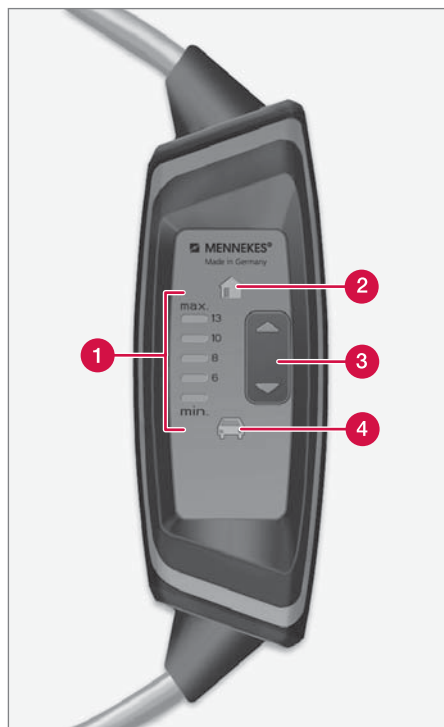
控制箱指示器及控制裝置。
