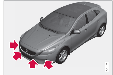
Sensorenverteilung vorn.
