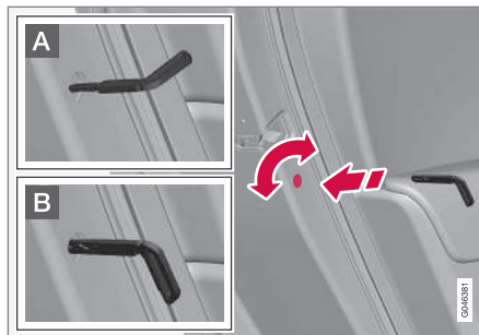
Manuelle Kindersicherung Nicht zu verwechseln mit dem manuellen Türschloss (S. 181).
