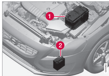
(1) Μπαταρία μίζας 17 (2) Εφεδρική μπαταρία
