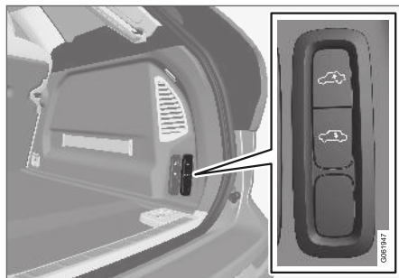
Reglage för höjning/sänkning av bilens bakparti.
