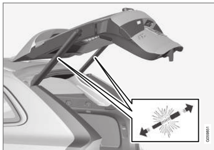
De förspända fjädrarna för den elmanövrerade bakluckan.
